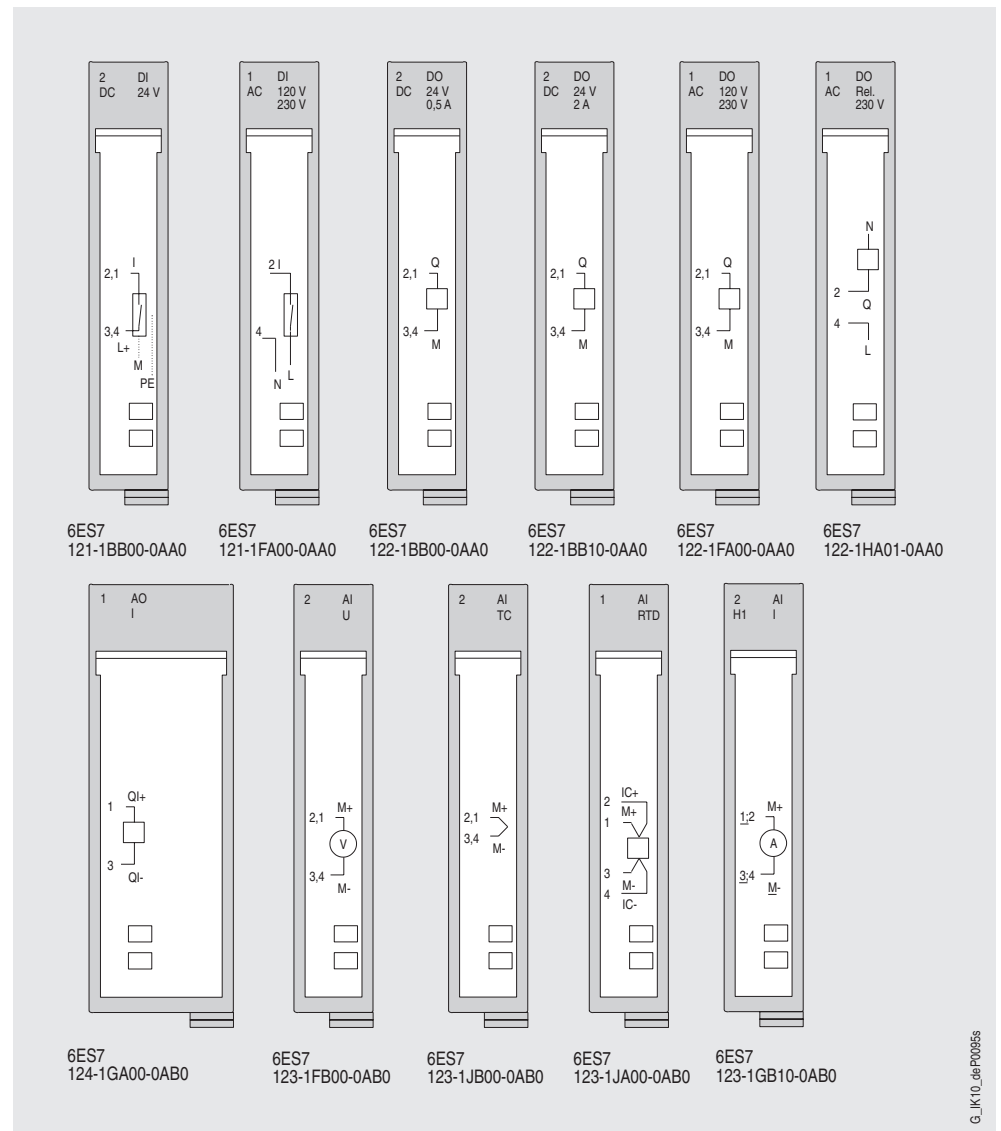
Bild 3/78 SIMATIC SC-Elektronikmodule
